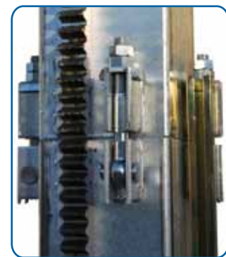
Unión de los tramos del mástil con tornillos de montaje rápido Mast sections assembling with quick-mounting screws
